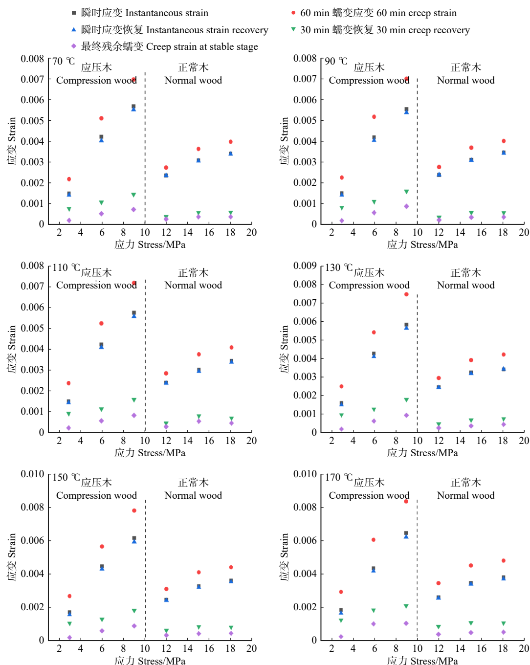
图6 不同应力水平下应压木和正常木早材试样拉伸蠕变参数(70~170 °C)
